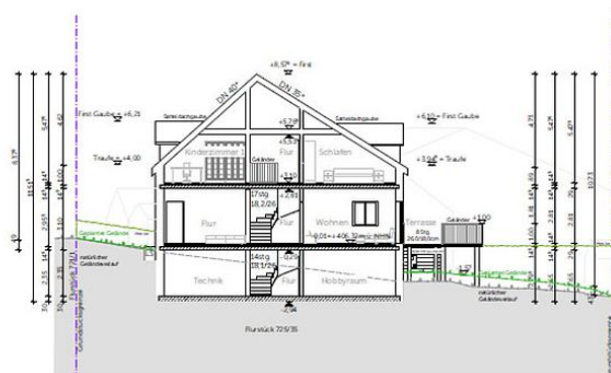
Schnitt H-H - M1:100
