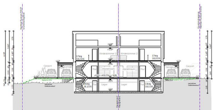
Schnitt A-A - M1:100
