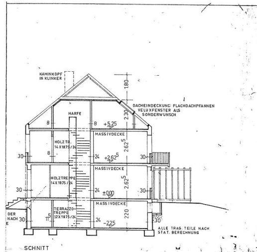
SCHNITT
